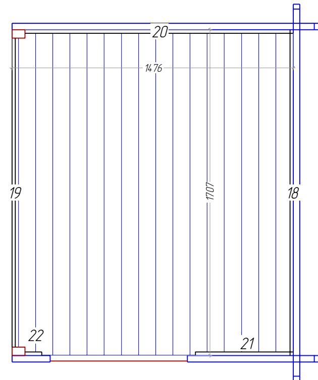
Fussboden
